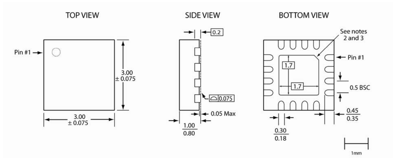
16-vqfn-3x3-QVC-2.0
