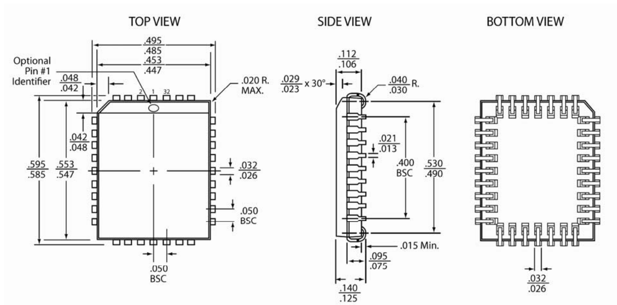
32-plcc-NH-3
