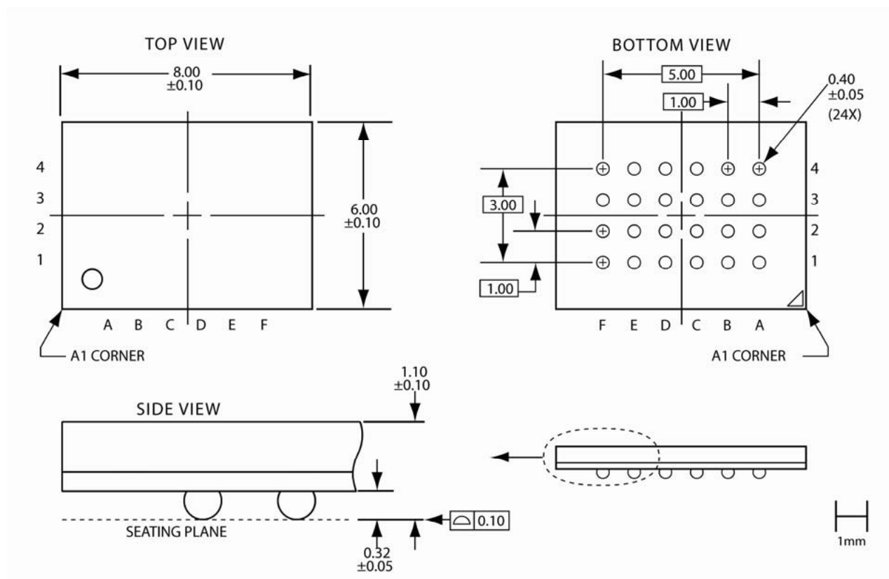
24-tbga-T4D-6x8-1.0
