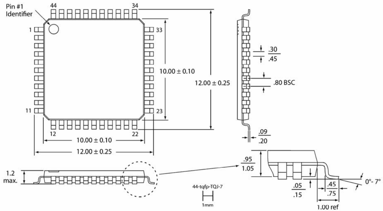
44-tqfp-TQJ-7
