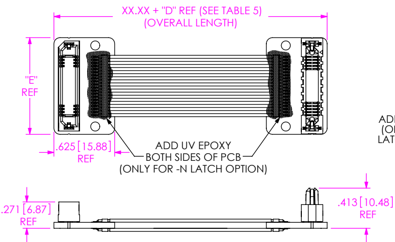
FIG 3 (ERCD-020-XX.XX-STL-TTR-1-N SHOWN)
