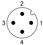
IO-Link
