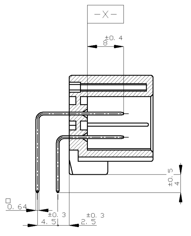
断面 A-A (SECT. A-A)
