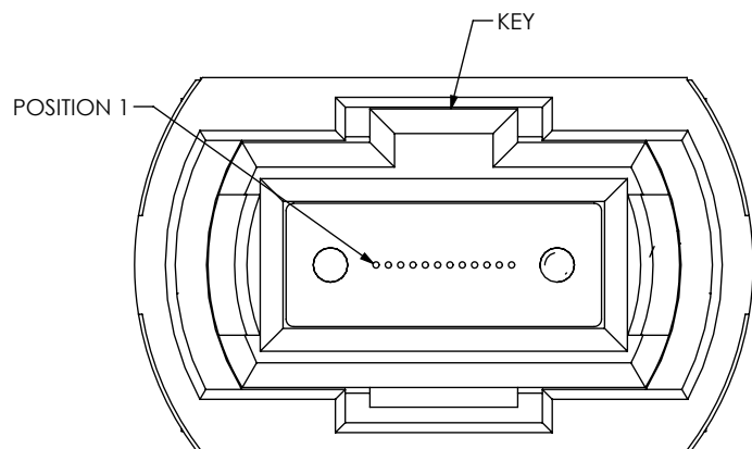
QSFP LOOPBACK
