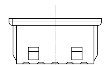
4 2, 3極ロック形状(1ロック) 4 4極以上ロック形状(2ロック) FIGURE OF 2, 3 CIRCUIT (1 LOCK) FIGURE OF MORE THAN 4 CIRCUIT (2 LOCKS)
