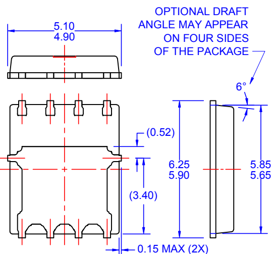
OPTION - B (PUNCHED TYPE)
