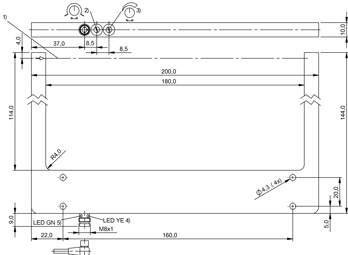
1) Optische Achse, 2) Empfindlichkeit, 3) Hell-/Dunkelschaltung, 4) Ausgangsfunktion, 5) Betriebsspannung
