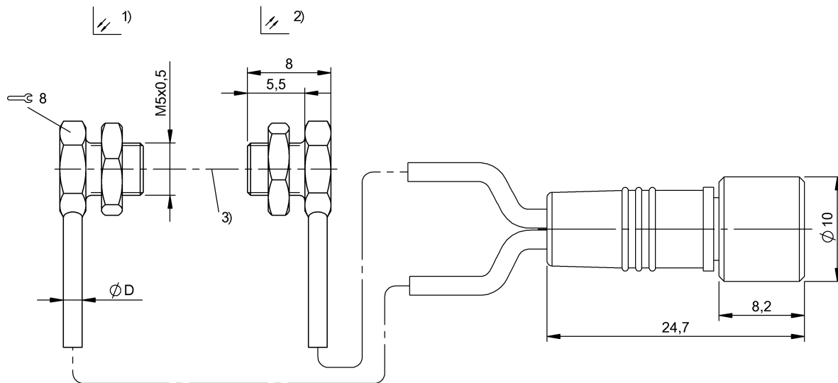
1) Sender, 2) Empfänger, 3) Optische Achse
