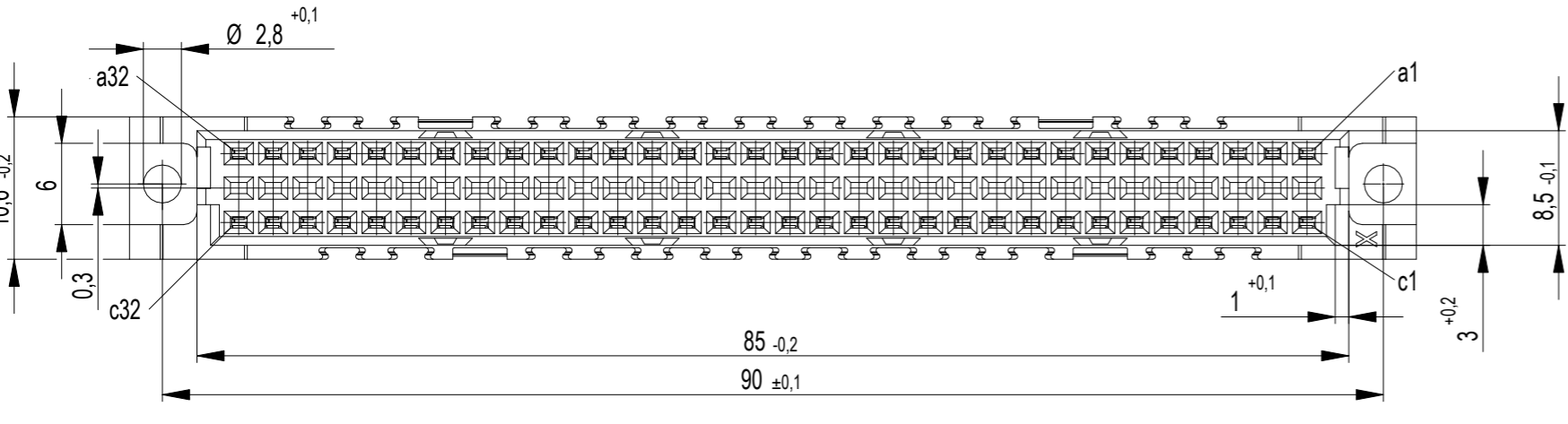
Bestückungsplan / contact layout
