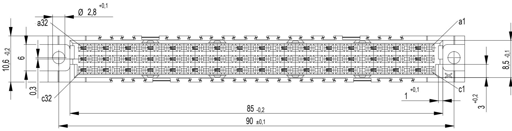
Bestückungsplan / contact layout
