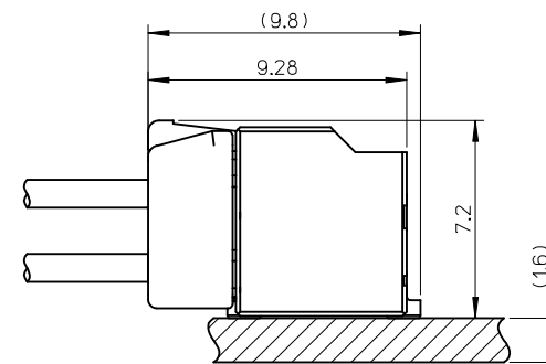
嵌合状態図 MATED CONNECTORS
