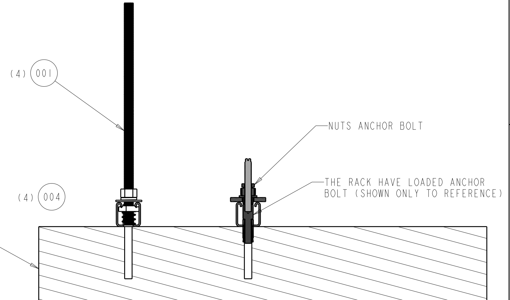
SECTION A-A SCALE 0.250
