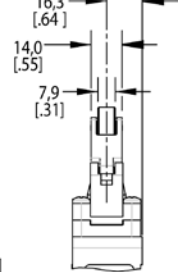
Figure 7. Top roller lever Abbildung 7. Oberer Rollenhebel Figura 7. Leva a rotella superiore Figure 7. Levier à galet supérieur Figura 7. Alavanca superior com roldana 그림 7. 상단롤러레버 Figura 7. Palanca con rodillo superior 图 7. 顶部滚轮操作柄
