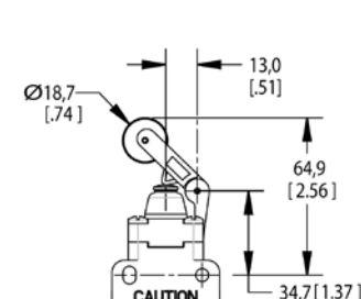
Figure 7. Top roller lever Abbildung 7. Oberer Rollenhebel Figura 7. Leva a rotella superiore Figure 7. Levier à galet supérieur Figura 7. Alavanca superior com roldana 그림 7. 상단롤러레버 Figura 7. Palanca con rodillo superior 图 7. 顶部滚轮操作柄
