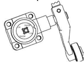
Abbildung 3: Bewegungsrichtung des seitlich angebrachten GSX-Drehkopfs ändern
