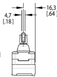
Figure 6. Top roller plunger Abbildung 6. Oberer Rollenstößel Figura 6. Pulsante a rotella superiore Figure 6. Poussoir à galet supérieur Figura 6. Êmbolo superior com roldana 그림 6. 상단롤러플런저 Figura 6. Êmbolo con rodillo superior 图 6. 顶部滚轮柱塞
